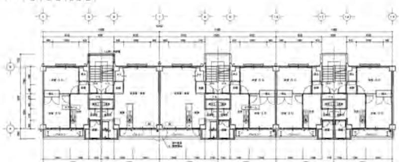
4 - 4階平面図 (改修後)
